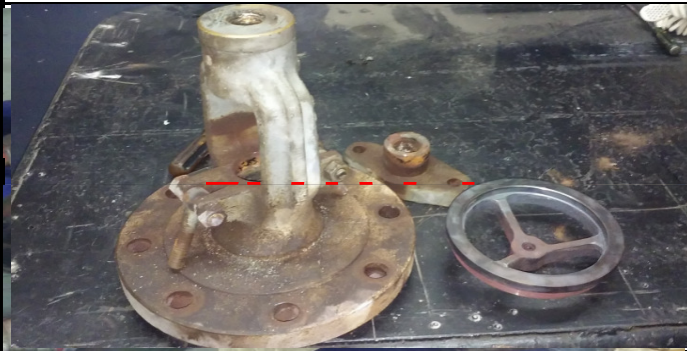
DESARME TOTAL DE VALVULA
